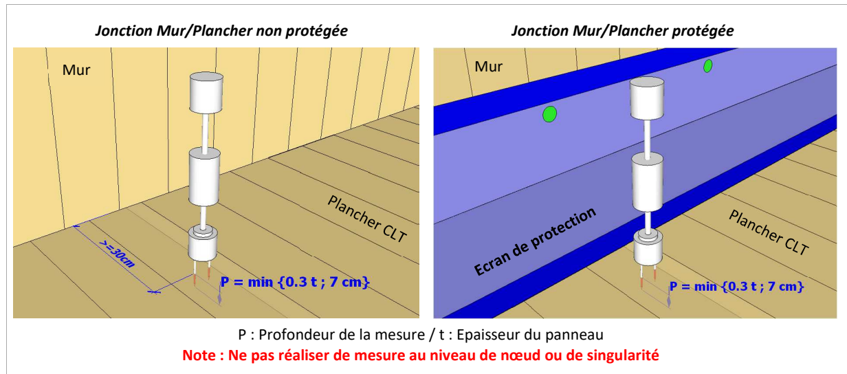
Figure 49 - Aperçu de mesure sur plancher CLT à la jonction plancher / Mur
