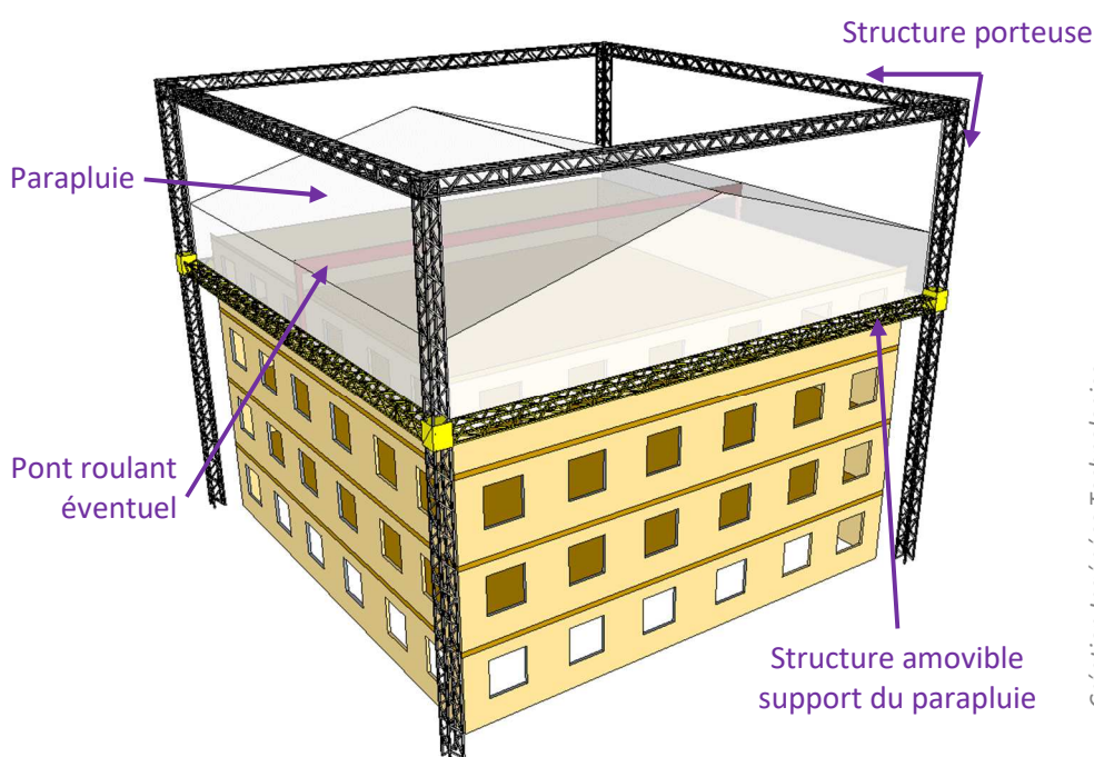
Figure 18 - Exemple de protection générale de type parapluie
