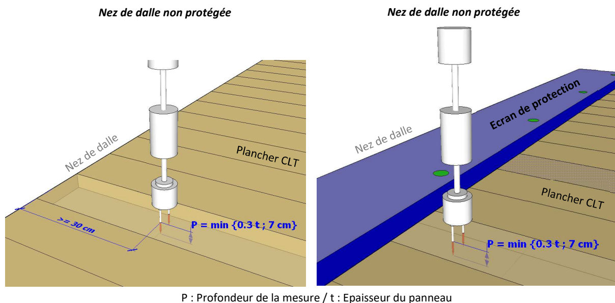
Figure 48 - Aperçu de mesure sur plancher CLT en nez de dalle
