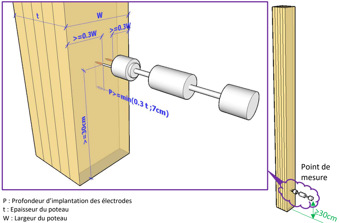
Figure 42 - Aperçu de mesure sur un poteau
