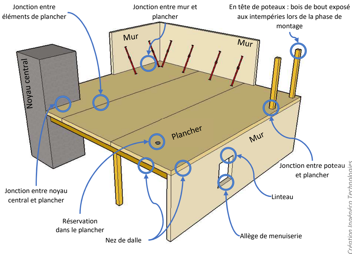
Figure 19 - Représentation des points singuliers pouvant potentiellement retenir l'eau en phase chantier
