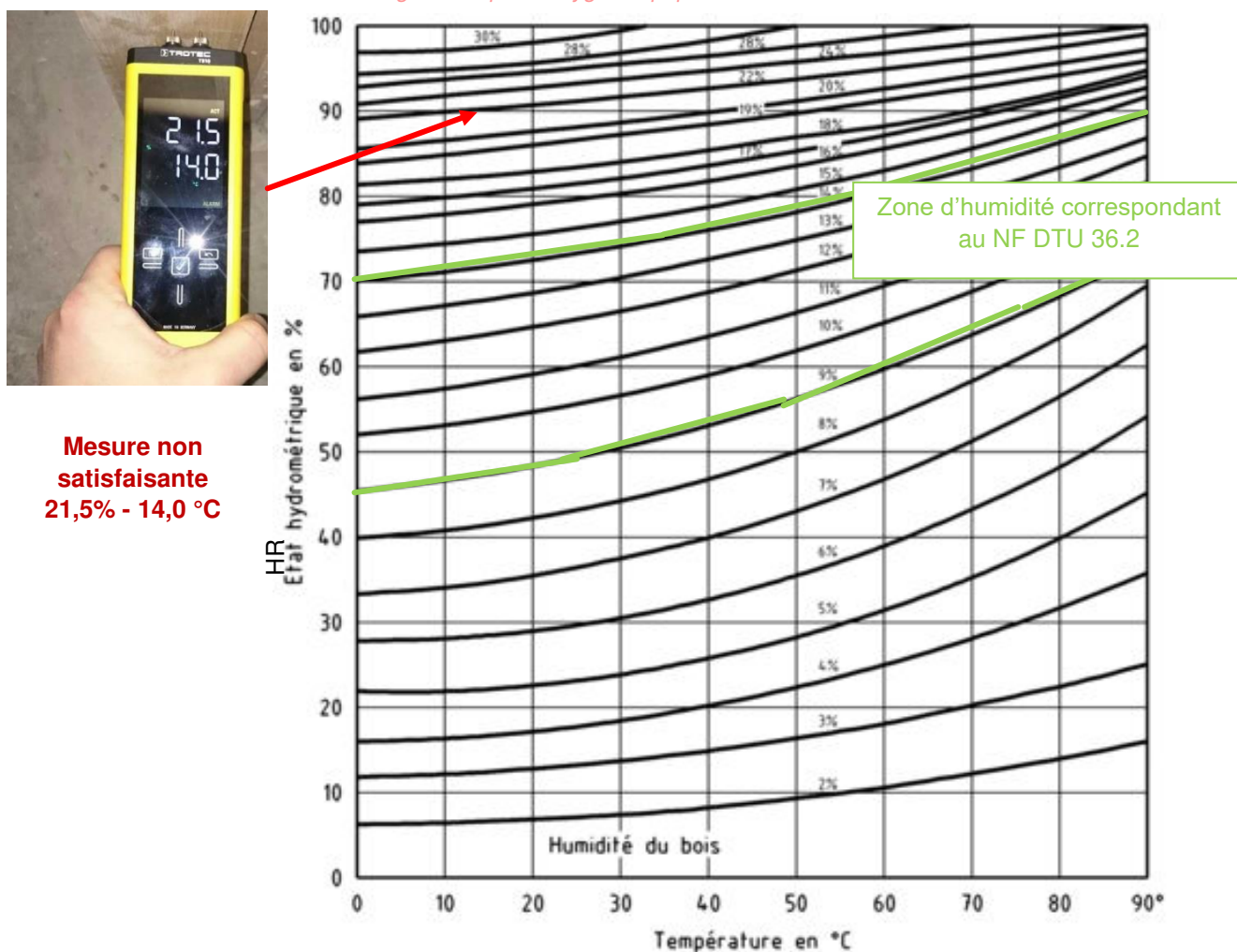
Figure 1 Equilibre hygroscopique des bois
